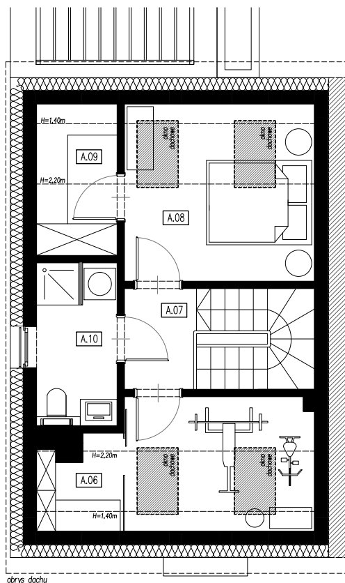
RZUT PODDASZA
