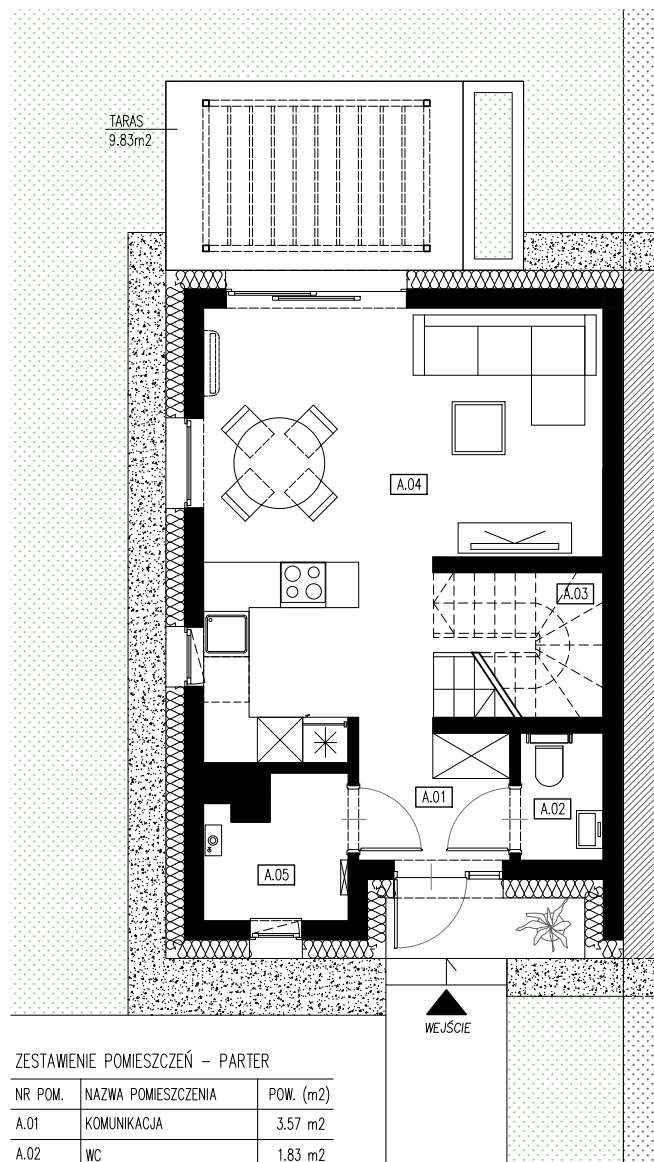
RZUT PARTERU
