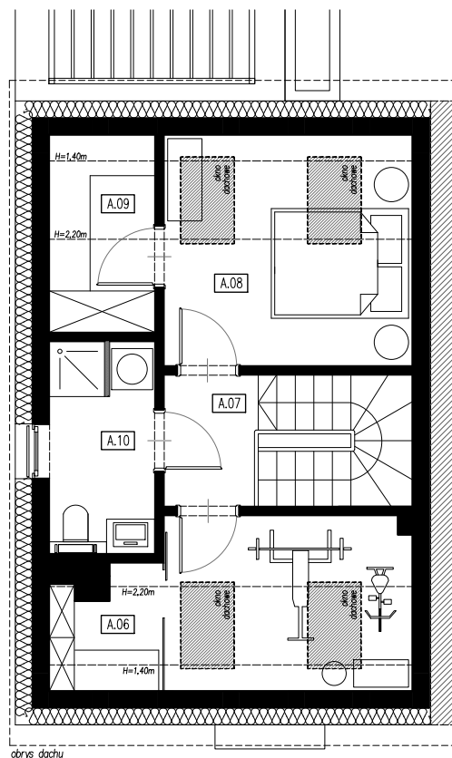
RZUT PODDASZA
